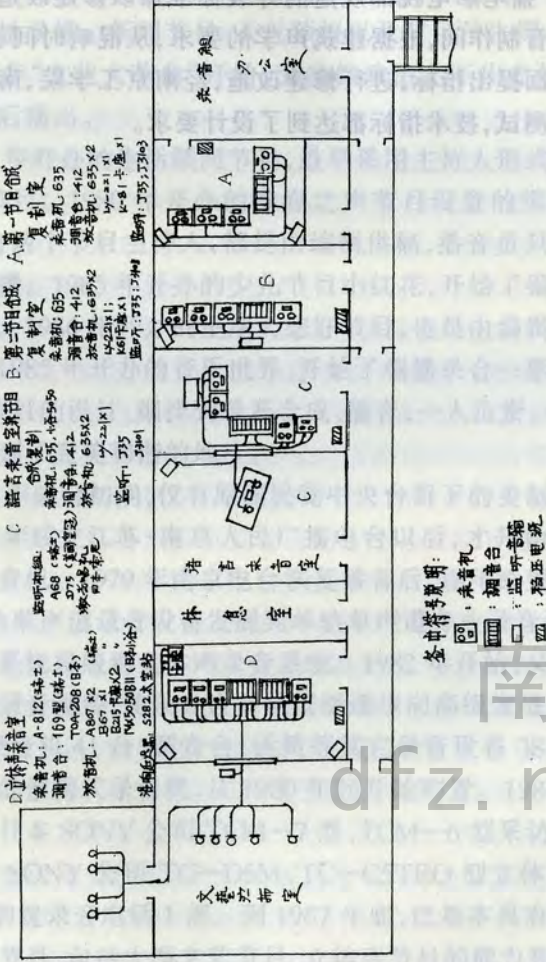
南京人民广播电台录音制作系统 设备配备平面位置图(老二楼)
