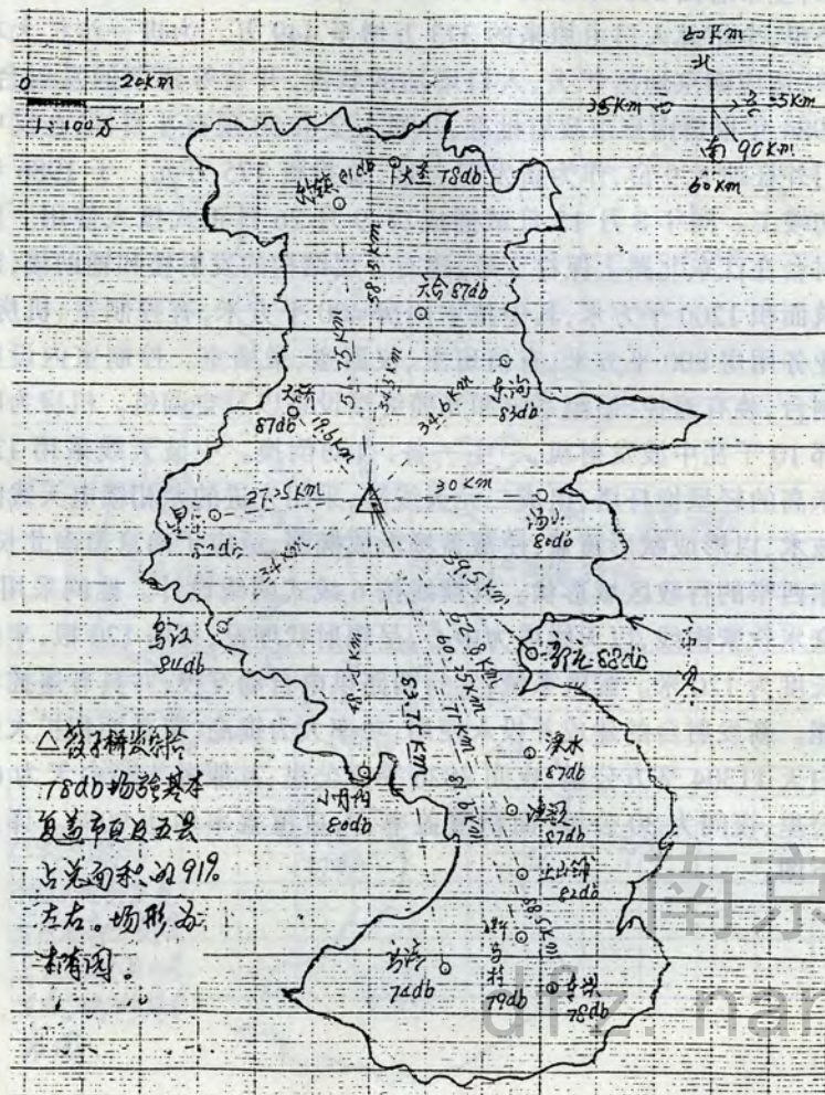
标称功率 10 千瓦场强覆盖示意图
